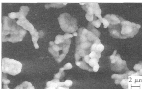
图 3 TAG:Ce 粉体颗粒的 SEM 照片
